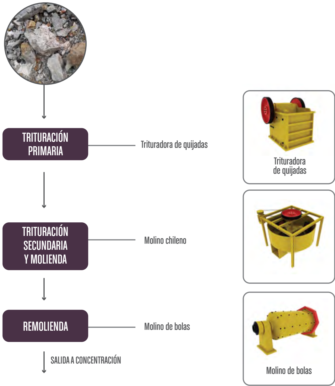
Figura 5.2: Diagrama de proceso de conminución (trituración y molienda) Fuente: Propia.
