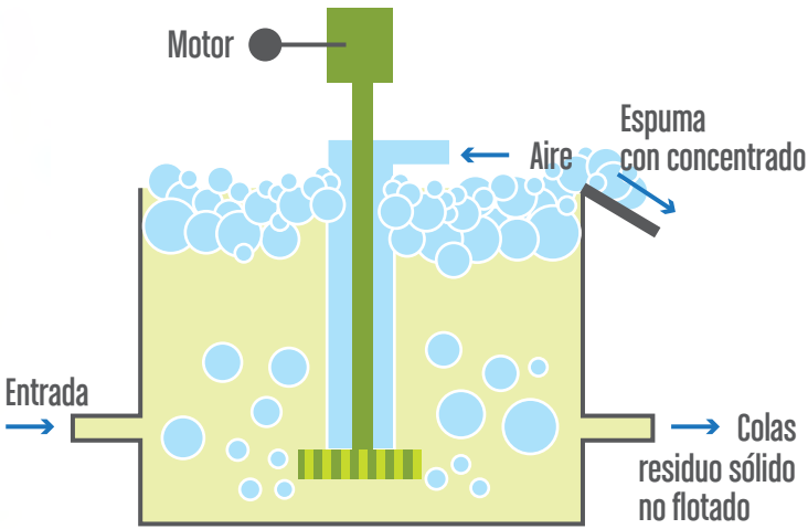
Figura 5.9: Diagrama de funcionamiento de una celda de flotación. Fuente: Propia.
