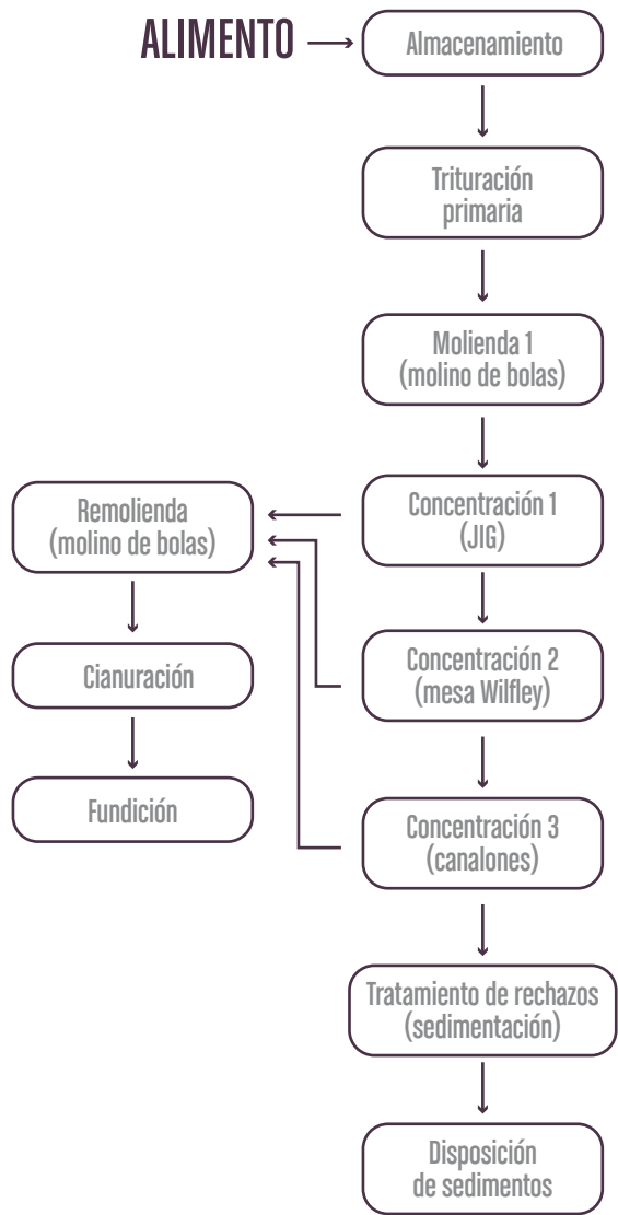
Figura 7.2: Diagrama de proceso de beneficio actual en la planta Gualconda municipio de Los Andes Sotomayor. Fuente: Propia.
