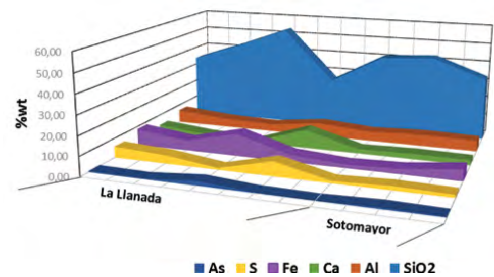
Figura 6.9: Composición elemental de Fe, S, Ca, Al, SiO2 para cabezas de proceso de La Llanada y Sotomayor. Fuente: Propia.
