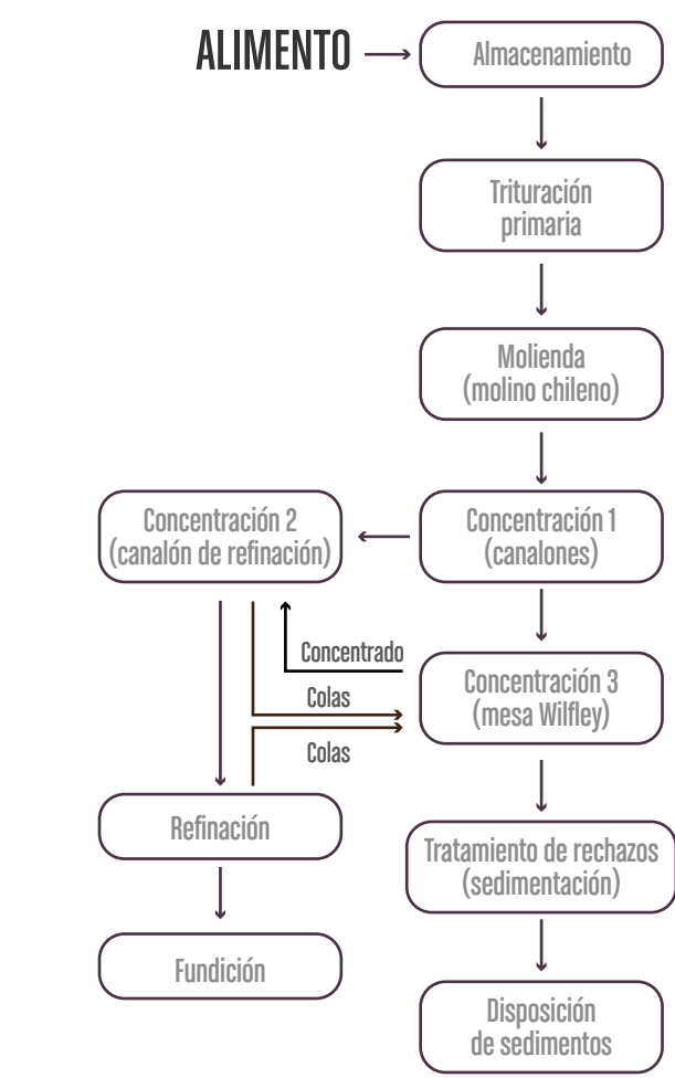
Figura 7.1: Diagrama de proceso de beneficio actual en La Llanada. Fuente: Propia.
