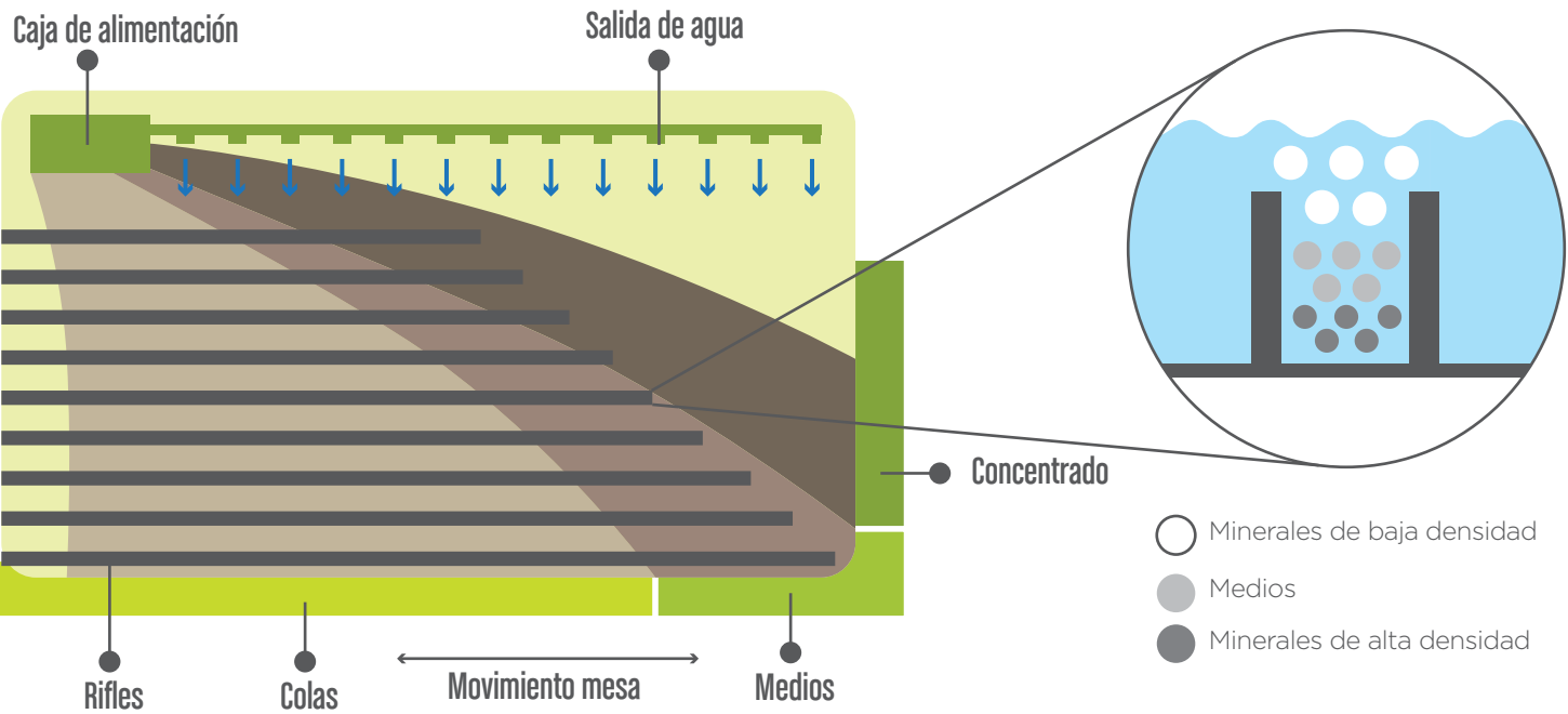
Figura 5.8: Diagrama de funcionamiento de una mesa de concentración gravimétrica. Fuente: Propia.
