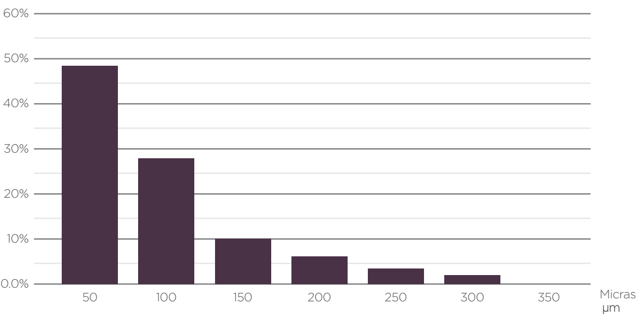
Figura 4.20: Distribución de oro en peso por rangos de tamaño zona de la Llanada. Fuente: Propia.
