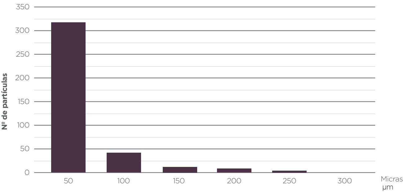
Figura 4.19: Tamaño de partícula de los grano de oro identificados en el sector de la Llanada. Fuente: Propia.
