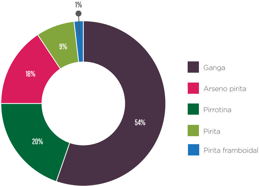
Figura 4.30: Composición mineralógica material de cabeza en la zona de La Llanada. Fuente: Propia.
