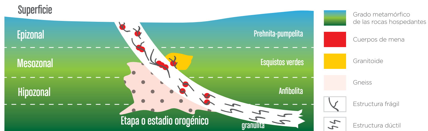
Figura 4.1: Depósitos orogénicos y los períodos geológicos. Fuente: Modificado de Goldfarb et al., (2001).
