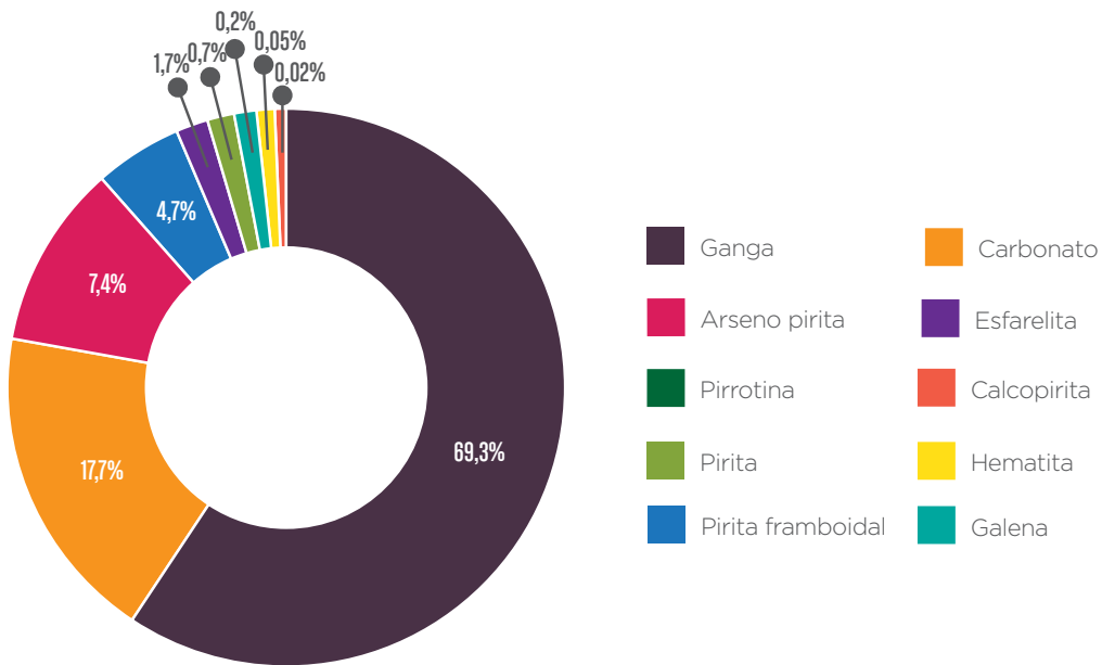
Figura 4.32: Composición mineralógica material de cabeza en la zona de Los Andes Sotomayor. Fuente: Propia.
