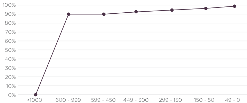
Figura 4.33: Grado de liberación material de cabeza en la zona de Los Andes Sotomayor. Fuente: Propia.
