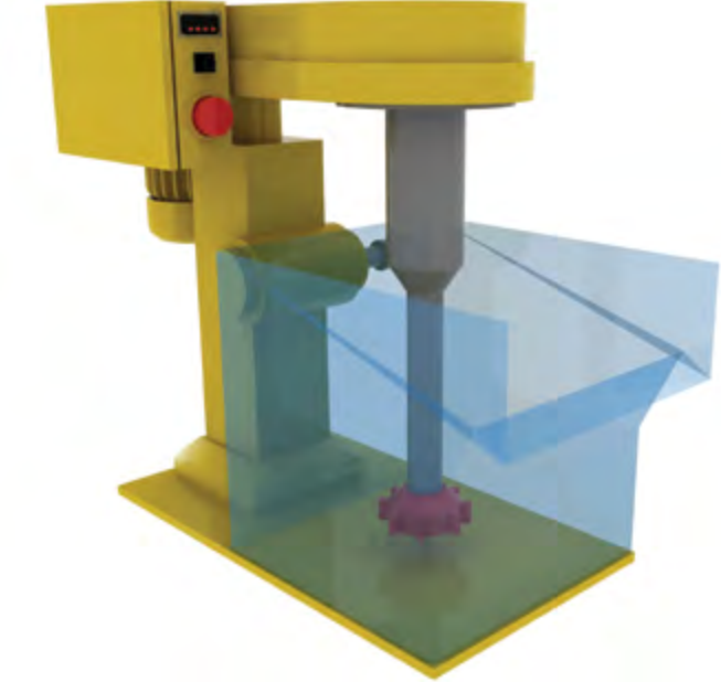
Fotografía 13: Modelo de celda de flotación industrial. Fuente: Propia.
