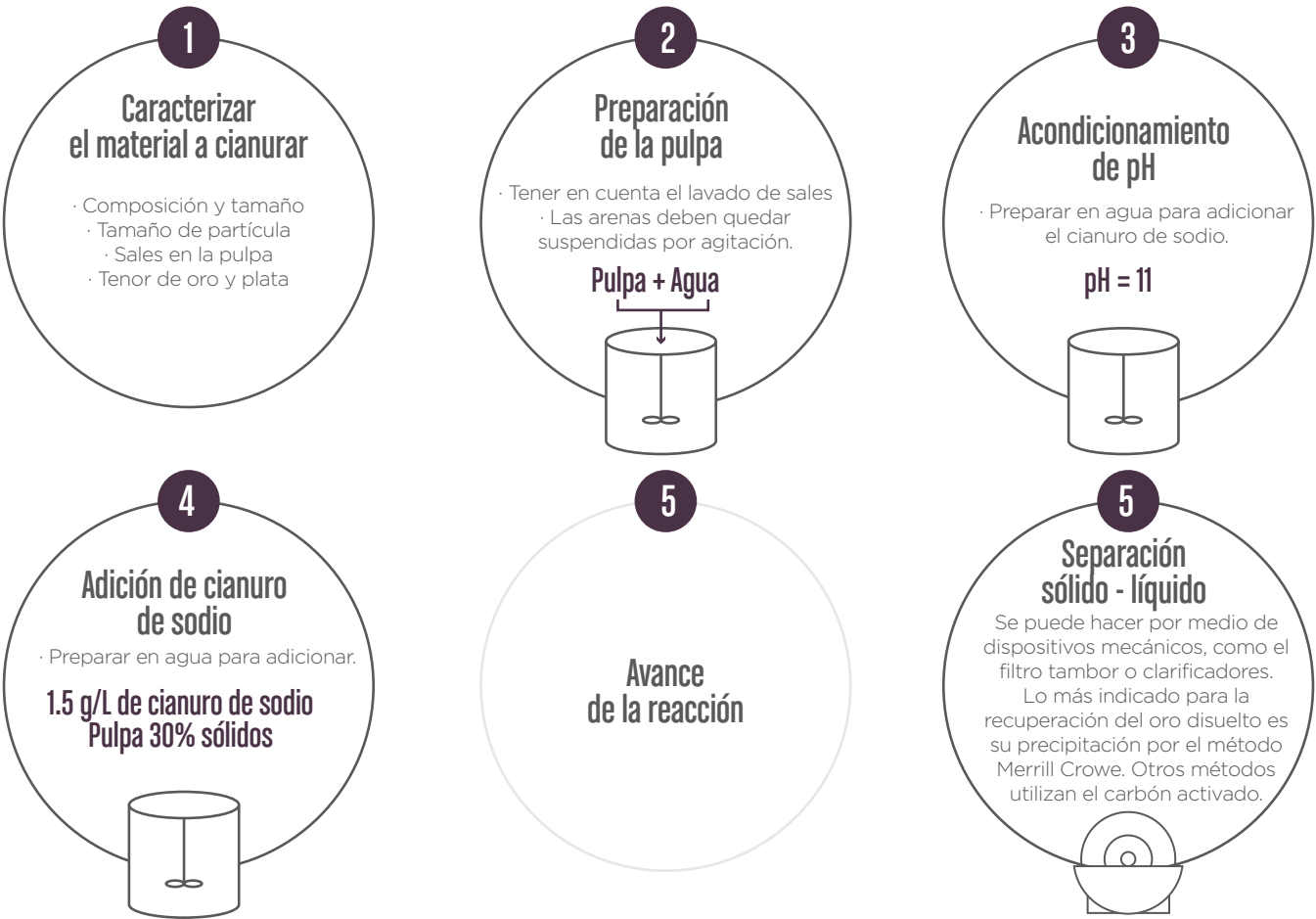
Figura 5.10: Diagrama de pasos a tener en cuenta para realizar el proceso de cianuración. Fuente: Propia.
