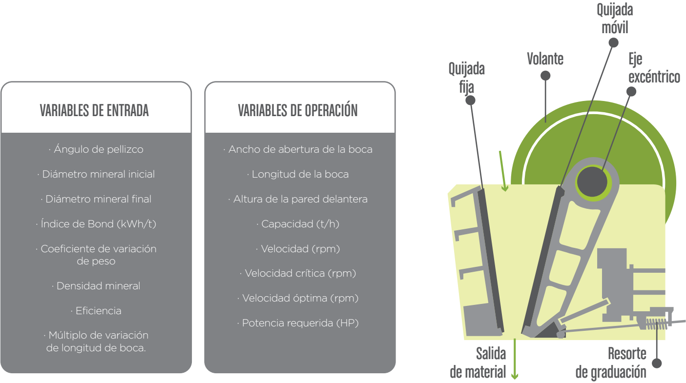
Figura 5.3: Diagrama de funcionamiento de la trituradora de quijadas. Fuente: Propia.
