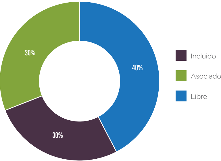
Figura 4.24: Ocurrencia de las partículas de oro observadas en la zona de Los Andes Sotomayor. Fuente: Propia.
