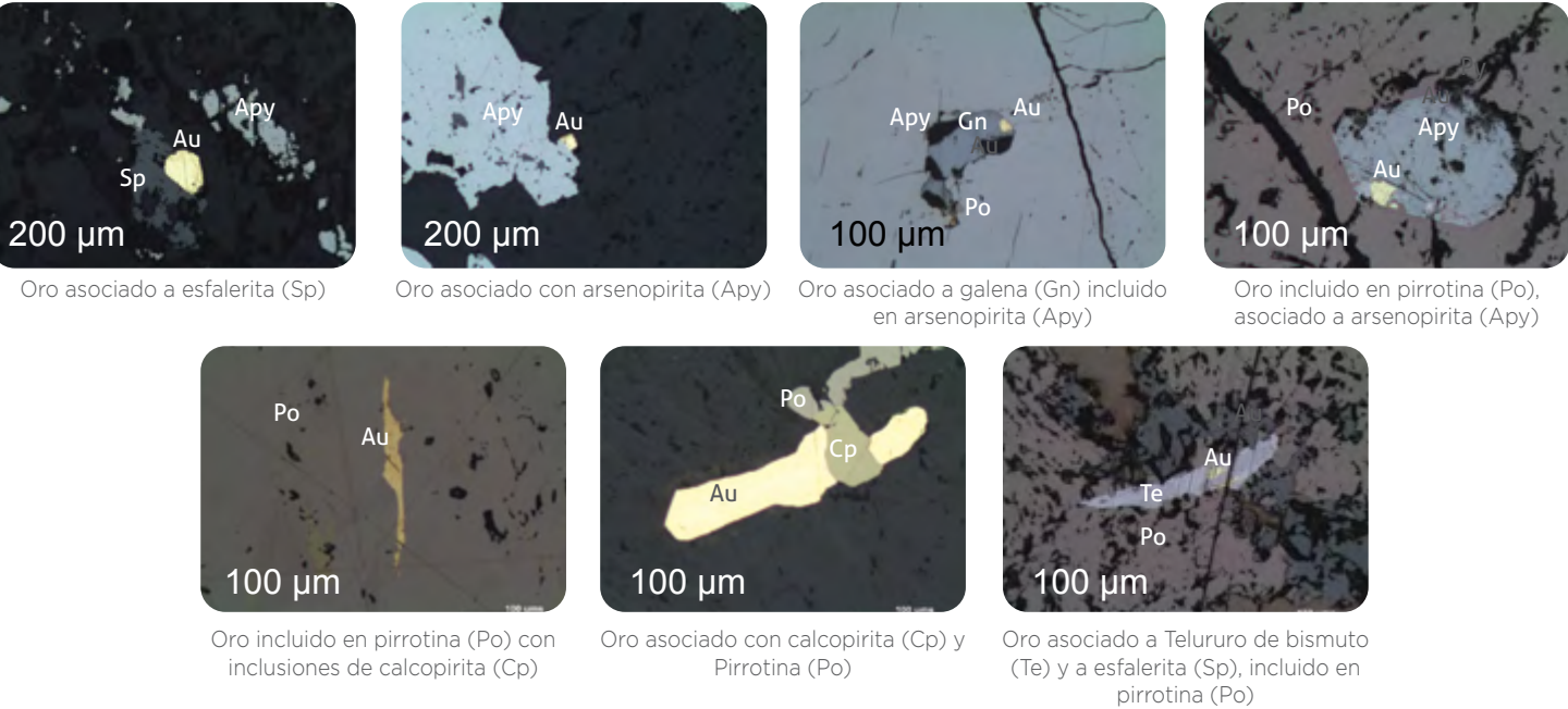
Figura 4.23: Imágenes de la ocurrencia de oro en La Llanada. Fuente: Propia.
