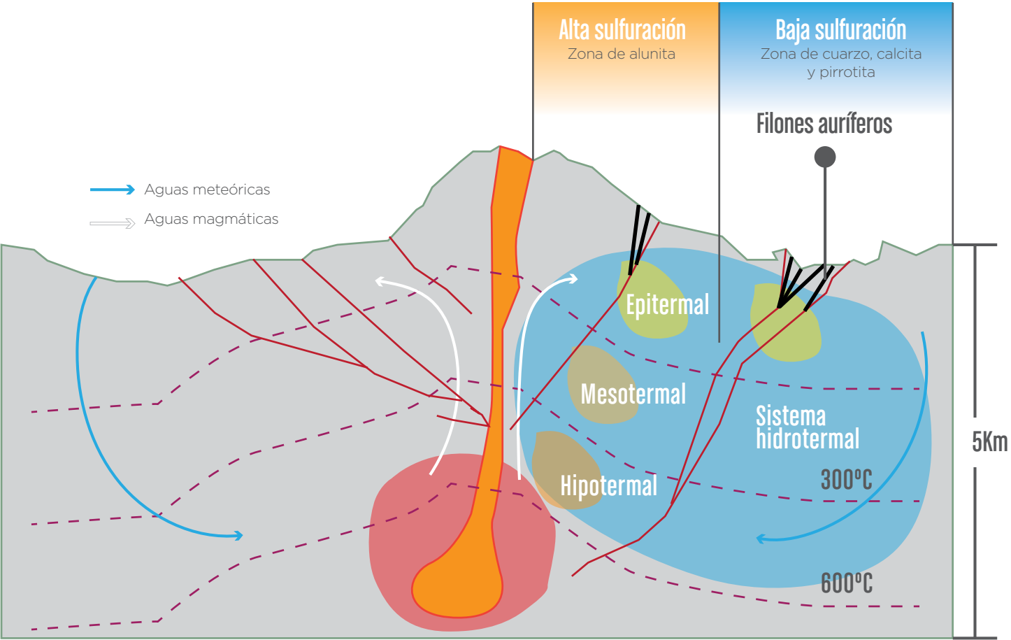
Figura 4.3: Perfil general de los depósitos auríferos de tipo hidrotermal (aproximación al ambiente de depósito aurífero en zona de minera). Fuente: Propia.
