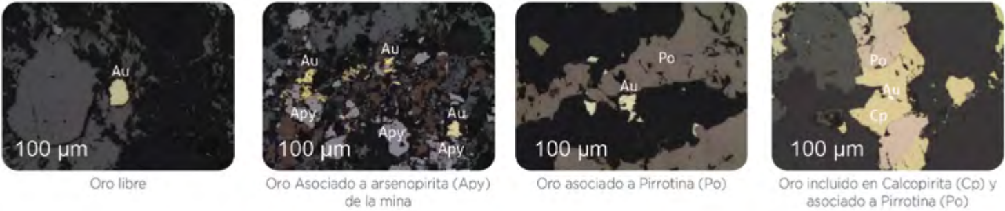
Figura 4.29: Imágenes de la ocurrencia de oro en Los Andes Sotomayor. Fuente: Propia.
