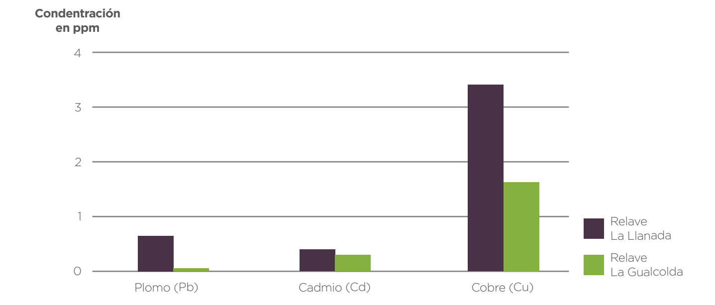
Figura 6.18: Composición elemental de relaves La Gualconda y La Llanada. Fuente: Propia.
